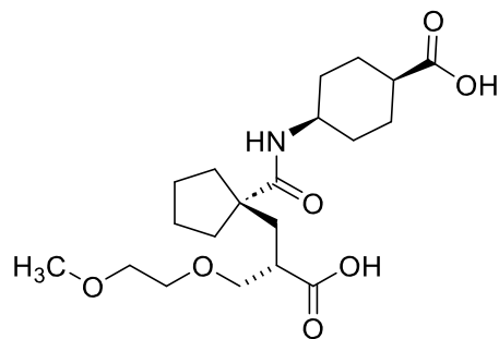
sandoksatriilaatti / sandoxatrilat
